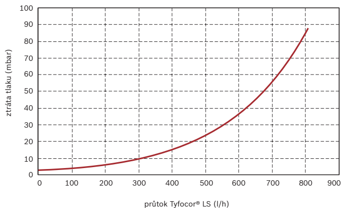
Graf tlakové ztráty kolektoru Xelios 2.5
