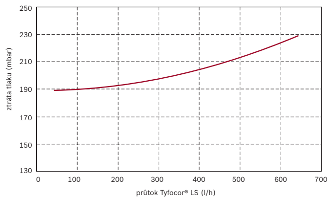
Graf tlakové ztráty kolektoru Xelios 2.0
